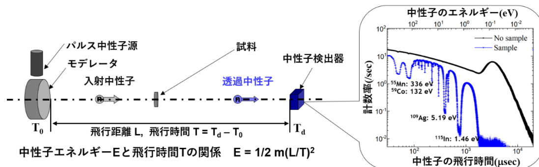
図1 NRTA法の概念図
